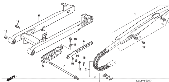
F-21 SWINGARM
