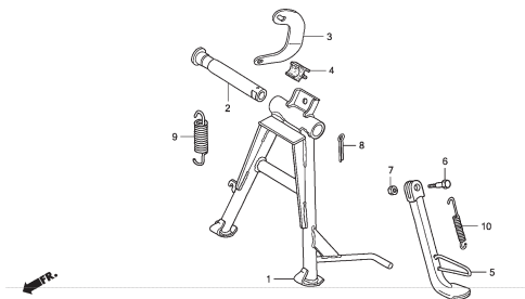
F20 STAND
