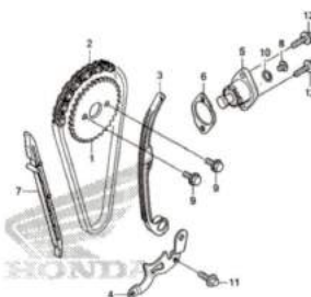
E-4 CAM CHAIN/TENSIONER
