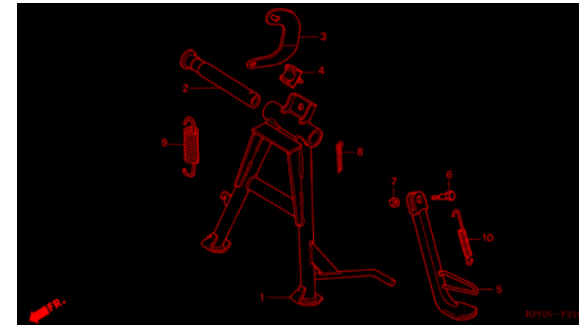
F-23 STAND
