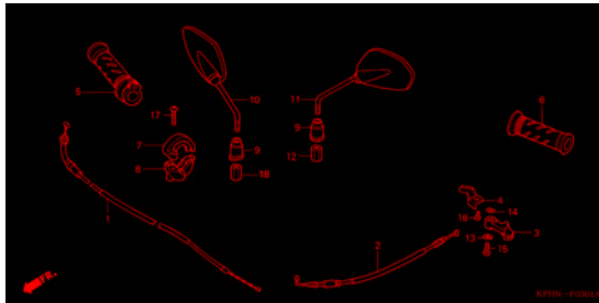
F-3-1 CABLE / MIRROR (Disk)
