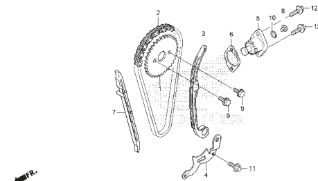
E-4 CAM CHAIN/TENSIONER
