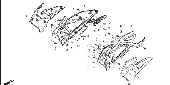
F-22-2 SHROUD(CB150RM)
