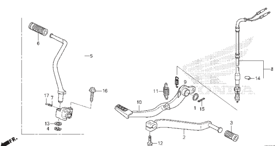
F-29 PEDAL
