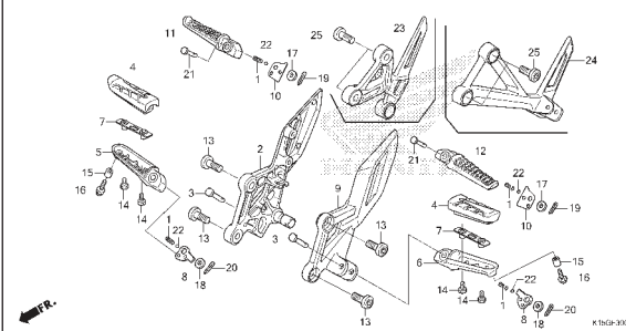
F-30 STEP
