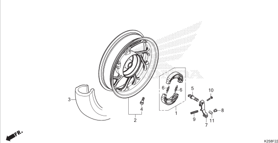
F-22-30 REAR WHEEL(ACB160CBT)
