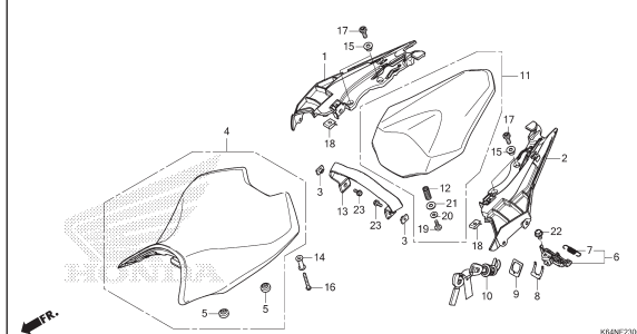
F-23 SEAT(CBR250S3L/S3M/S3AL/S3AM)
