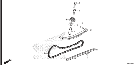
E-5 CAM CHAIN/TENSIONER
