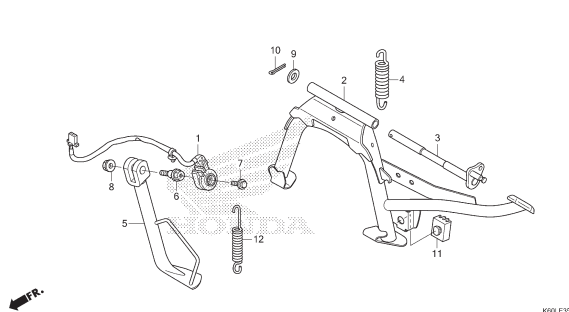
F-35 STAND
