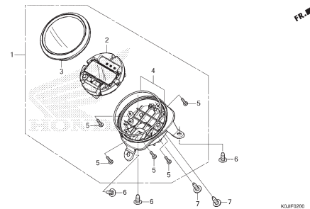
F-2 METER
