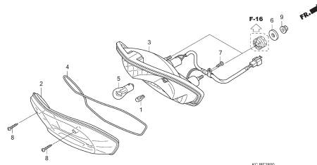
F-28 TAILLIGHT (Tiger Revo)
